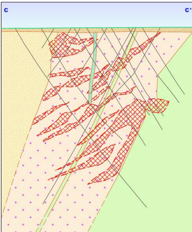
Figure 3c: Caloma cross section 6394305mN MGA
